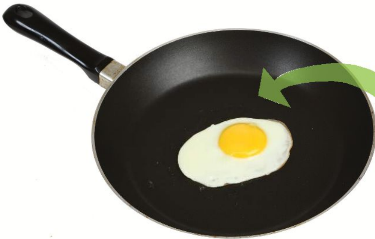
تَغْيِيرُ كِيمِيَاءِيٍّ
